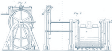
№ 16,082. H. BESSEMER, МАШИНЫ ДЛЯ ПЛАВКИ ЖЕЛЕЗА. Patented Nov. 11, 1856.
